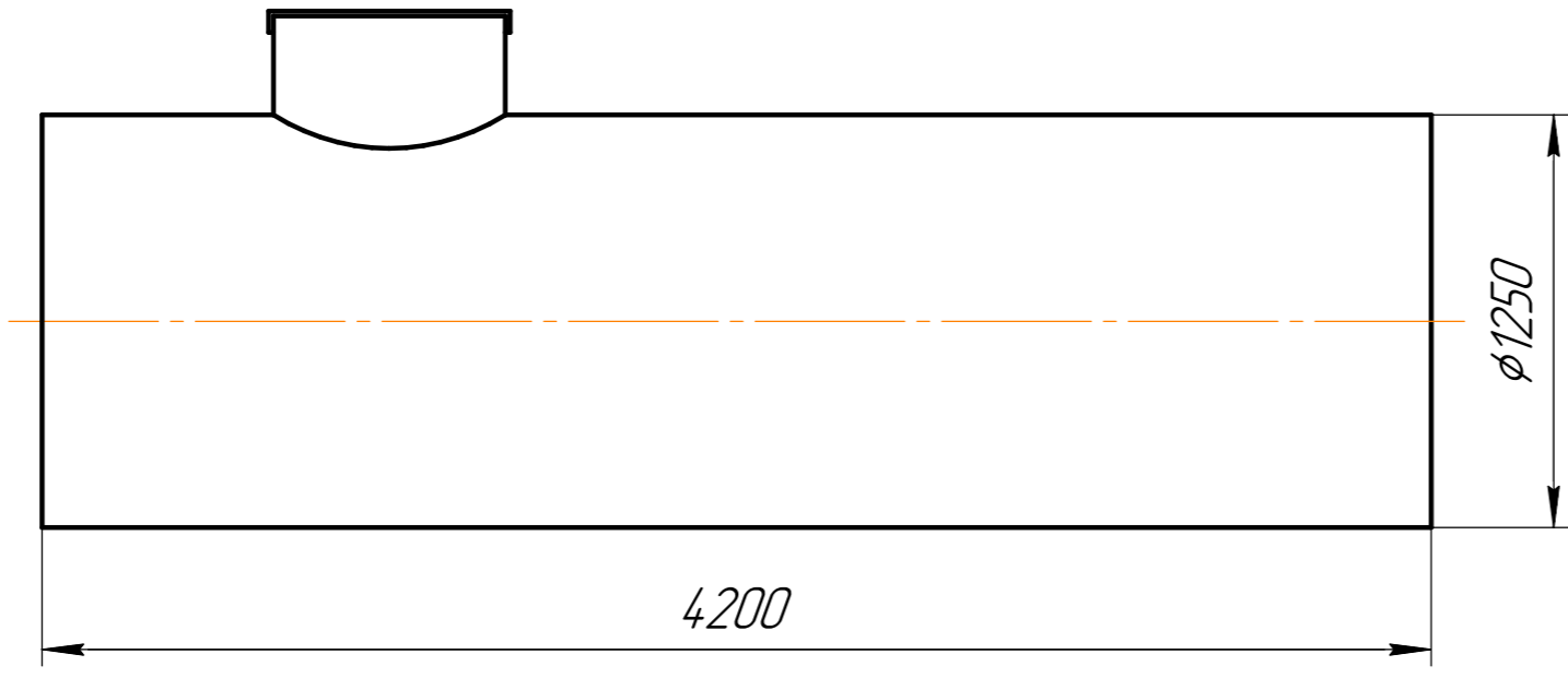
Разрез 1-1
