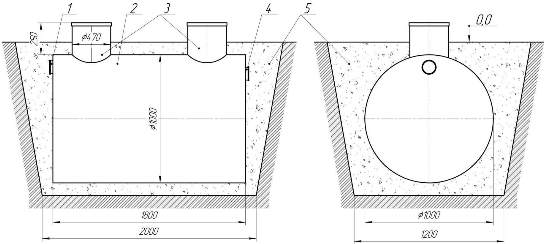
Рисунок А.1 Монтаж Энергонезависимого септика «Дрена-БИО 4» на подготовленное песчаное основание
