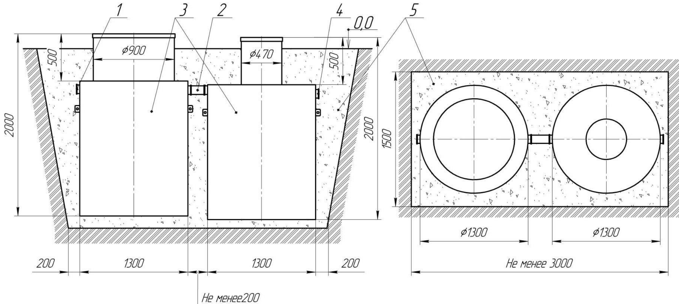
Рисунок А.1 Монтаж ЛОС «Биосфера 15» на подготовленное песчаное основание
