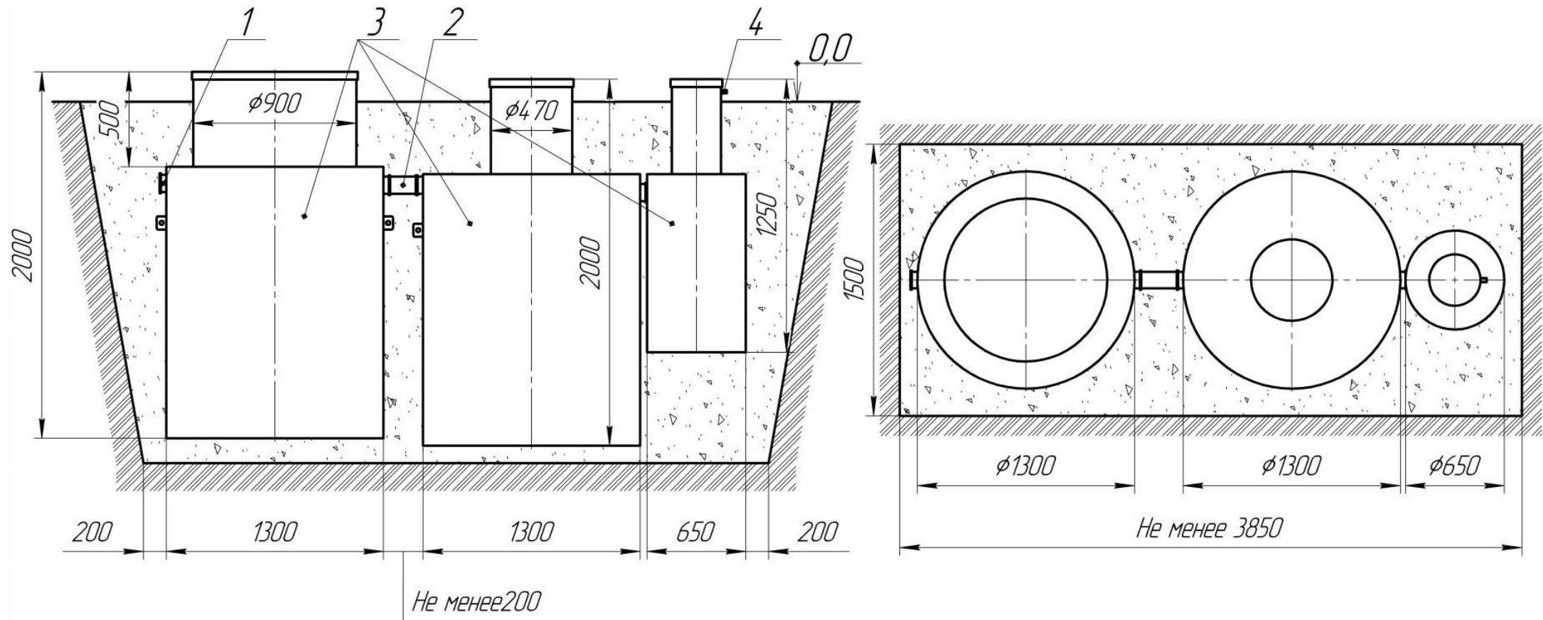
Рисунок А.2 Монтаж ЛОС «Биосфера 15 ПР» оборудованной принудительным водоотведением на песчаное основание
