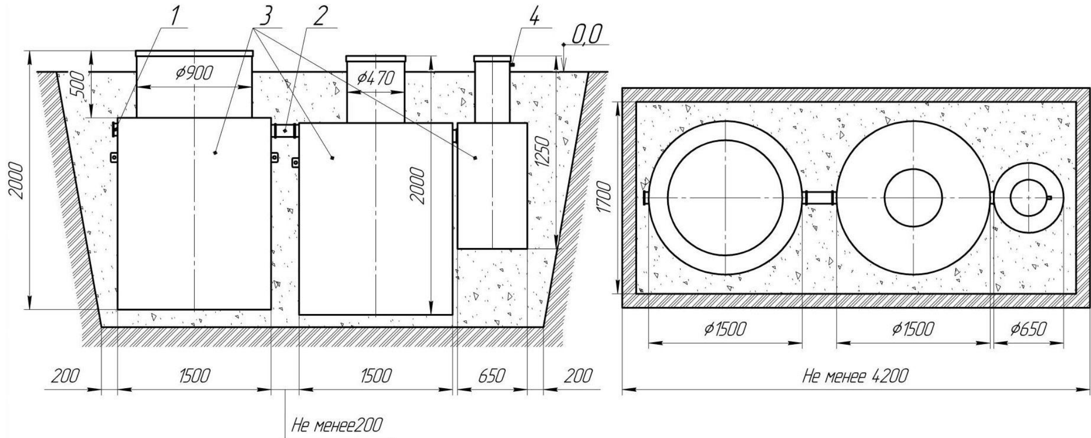
Рисунок А.2 Монтаж ЛОС «Биосфера 20 ПР» оборудованной принудительным водоотведением на песчаное основание
