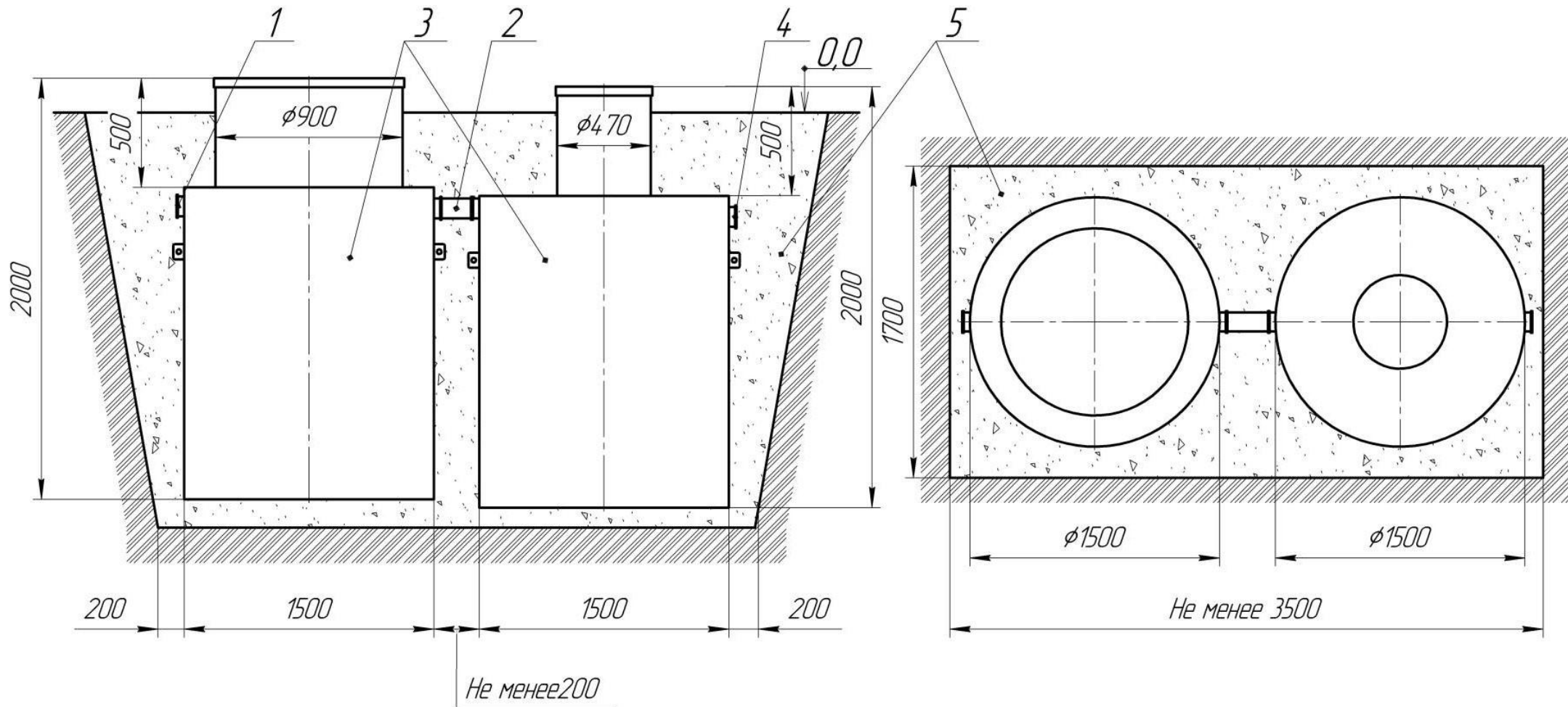
Рисунок А.1 Монтаж ЛОС «Биосфера 20» на подготовленное песчаное основание
