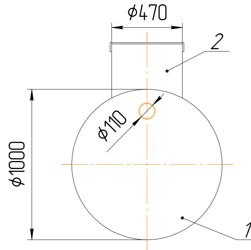
Вид спереди
