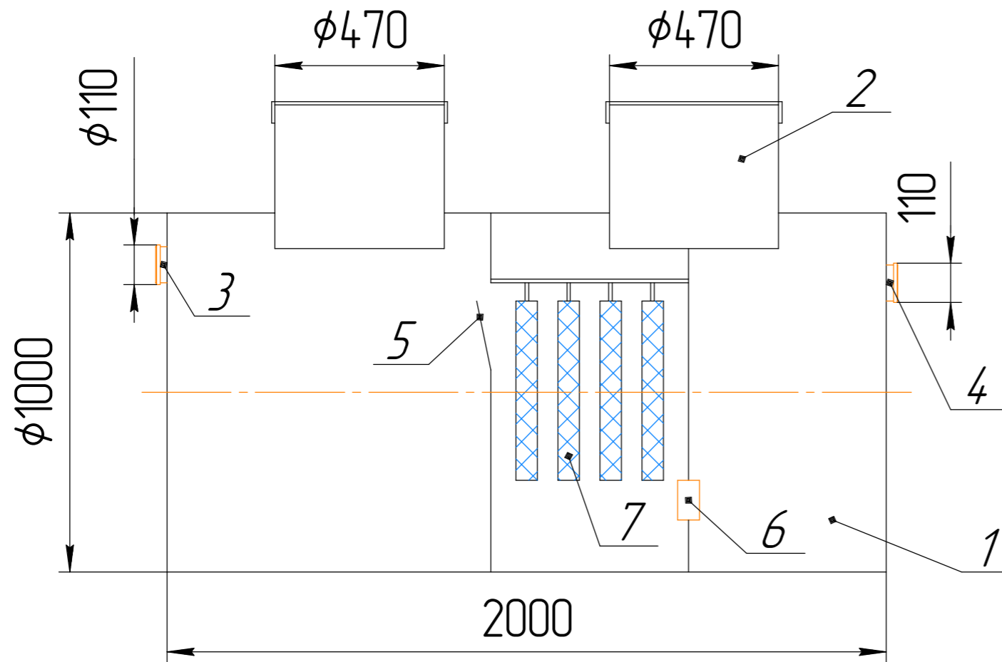
Разрез
