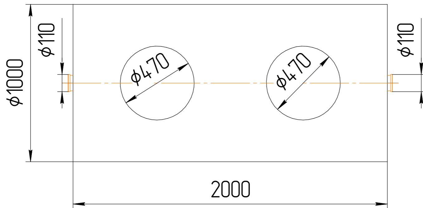
Вид сверху
