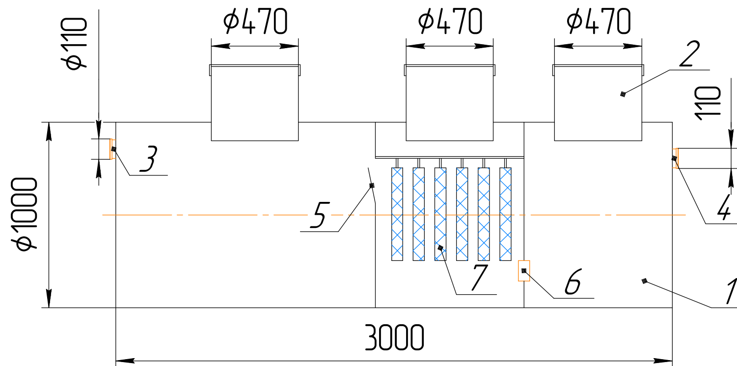
Разрез
