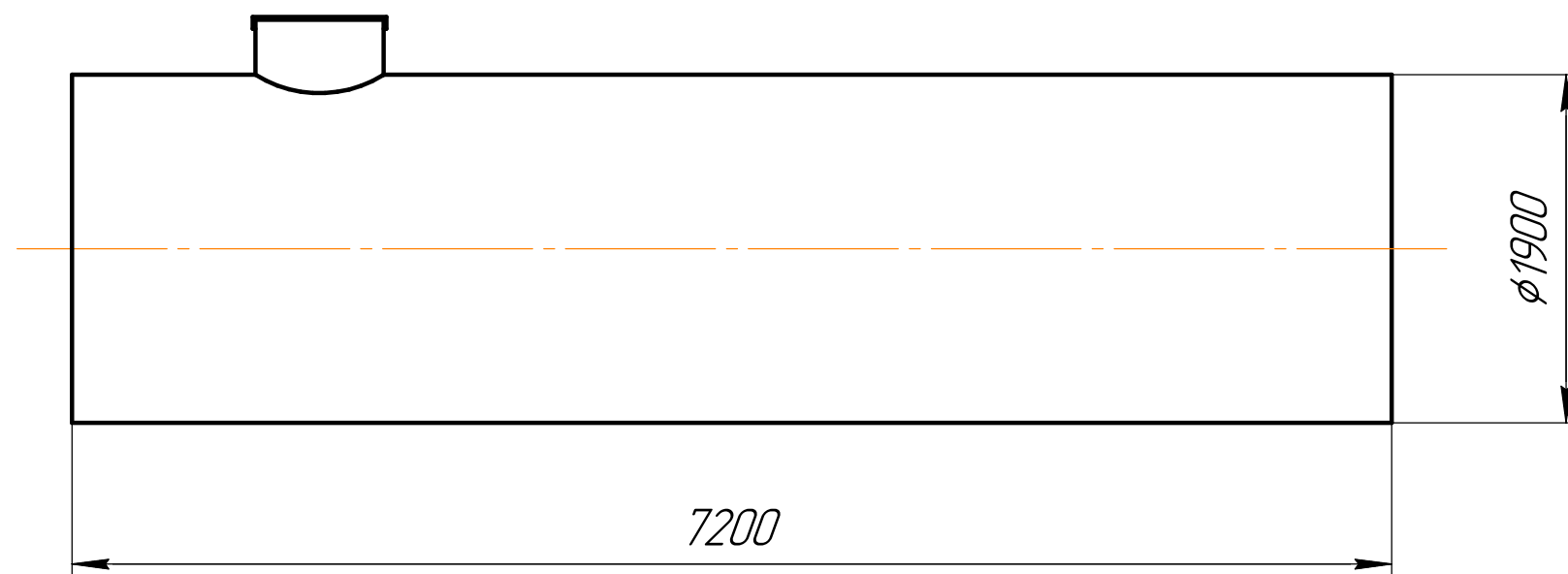
Разрез 1-1
