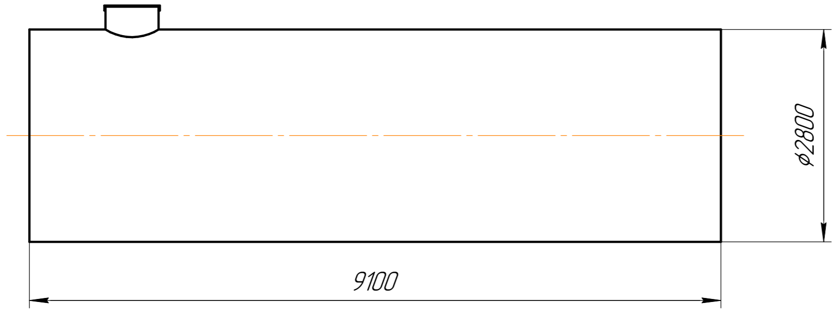
Разрез 1-1
