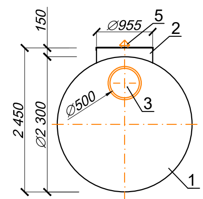
Вид спереди
