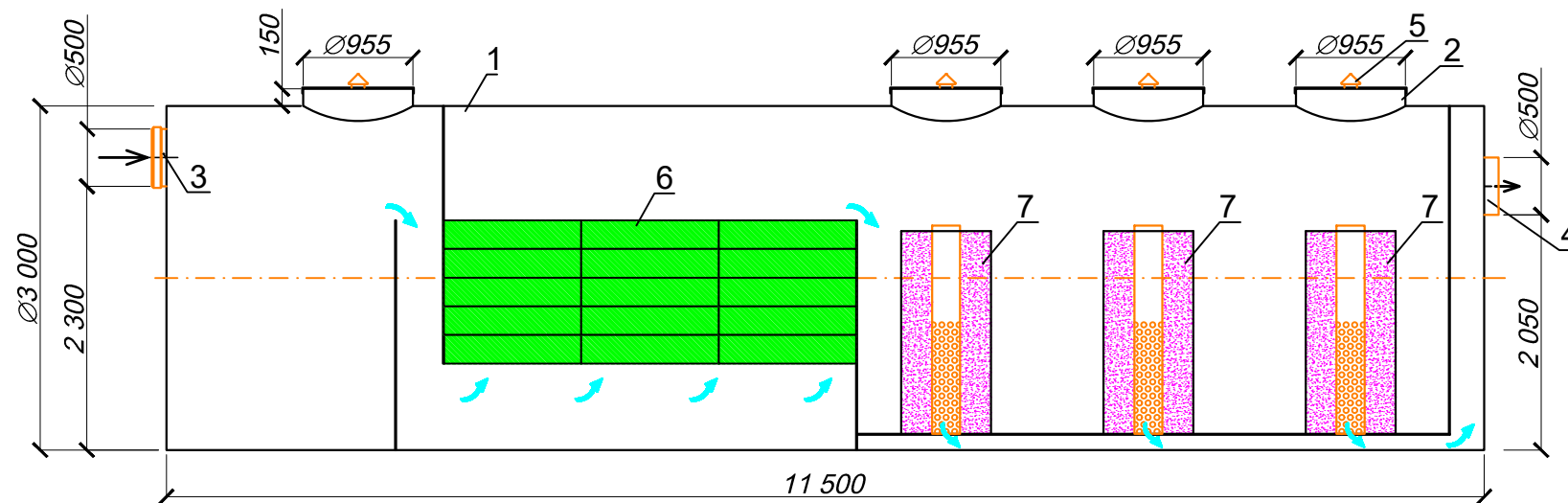
Разрез 1-1
