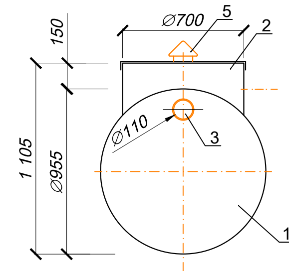
Вид спереди
